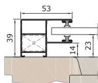
Vodící lišta KE53V pro renovace
