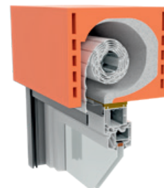
ROLL S šachta
