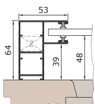
Vodící lišta KD53V
