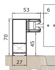
Vodící lišta ED53V
