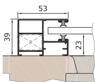
Vodící lišta KF53V
