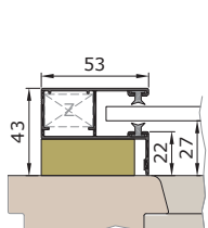
Termicky oddělená vodící lišta K53VT
