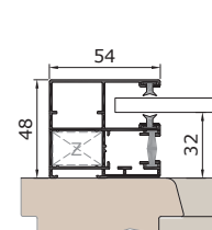
Vodící lišta KR54V
