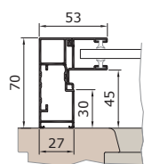
Vodící lišta KD53SA
