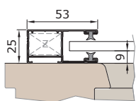
Vodící lišta K53V
