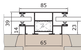
Sloupek s vodící lištou K85V
