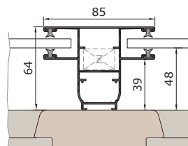
Sloupek s vodící lištou KD85V
