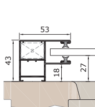
Vodící lišta KA53V
