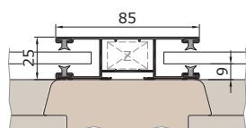
Sloupek s vodící lištou K85V
