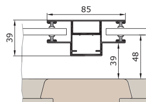
Sloupek s odsazenou vodící lištou
