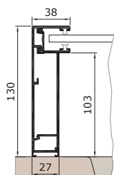
Vodící lišta KH38SA
