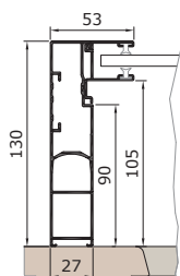
Vodící lišta KH53SA
