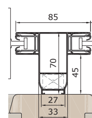
Sloupek s ED85V
