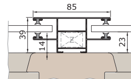
Sloupek s vodící lištou KE85V
