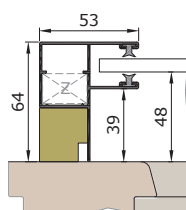
Termicky oddělená vodící lišta K53VT
